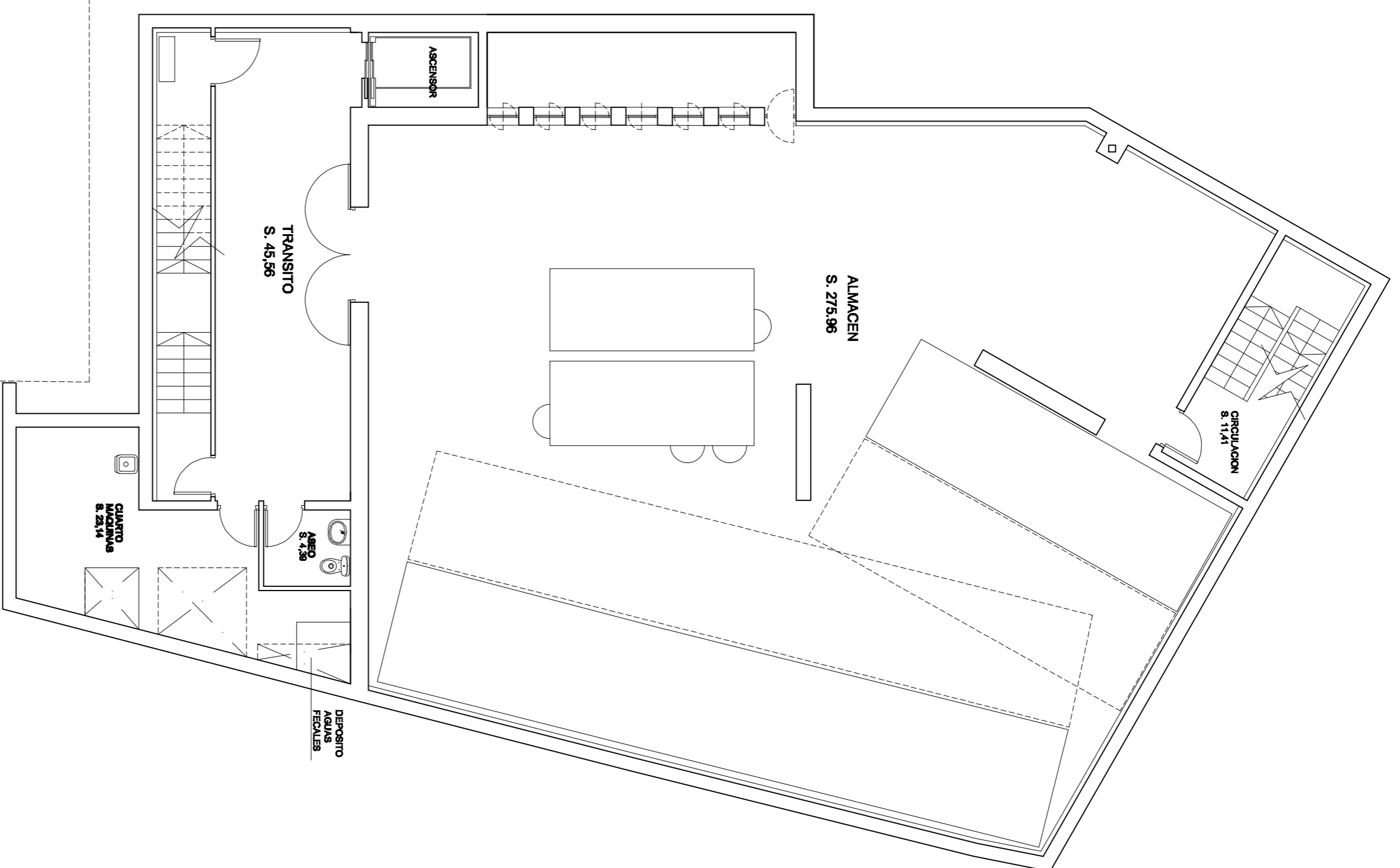
Planta nivel -2
