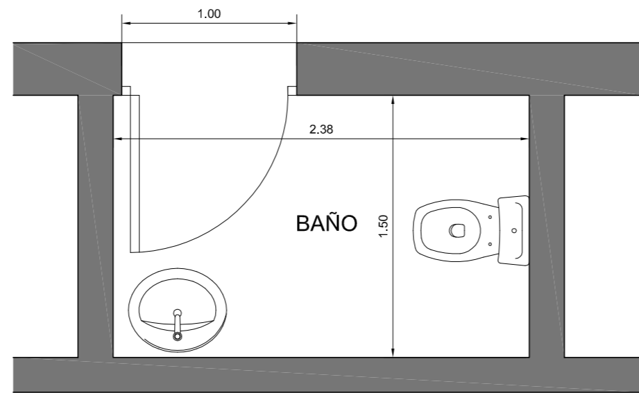
BAÑO ADAPTADO ESTADO ACTUAL ESC 1/30
