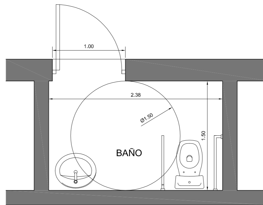
BAÑO ADAPTADO ESTADO ADAPTADO ESC 1/25
