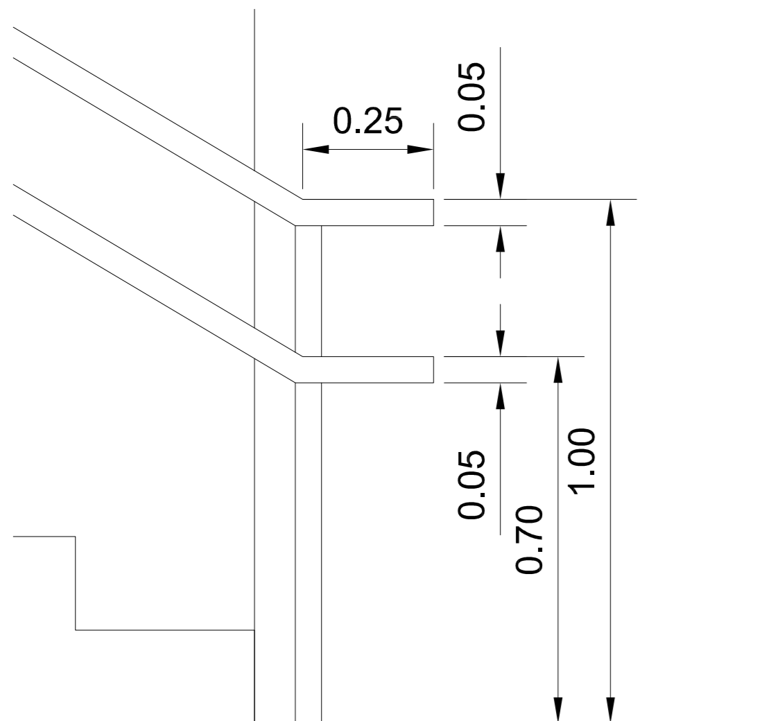
DETALLE BARANDILLA ESC 1/10
