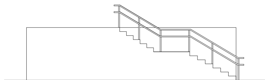
DETALLE BARANDILLA ESC 1/10
